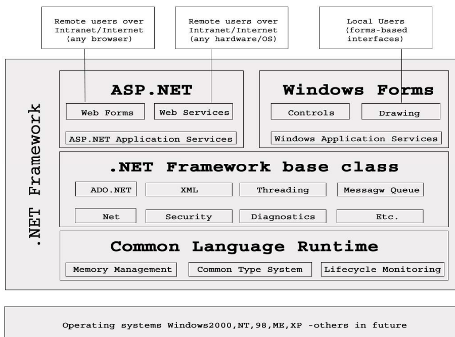
รูปที่ 7-2 องค์ประกอบ .NET Framework
